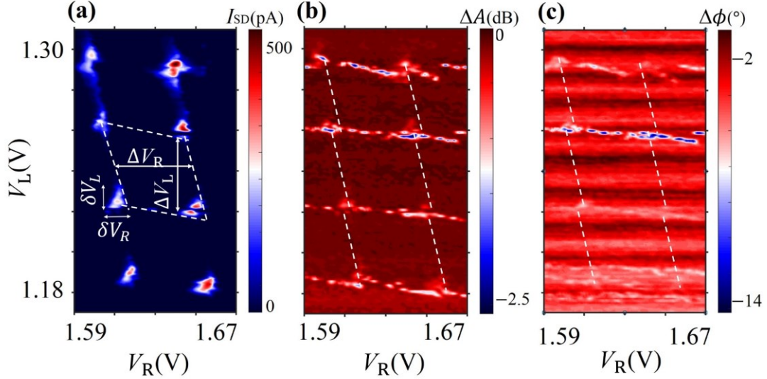
图 4.6 (a) 源漏偏压 V_{SD} = 1.5 \text{ mV} 时，双量子点直流运输的电荷稳定性相图，空穴在量子点中和源漏之间隧穿用白色虚线表示。 \delta V_L 和 \delta V_R 对应偏压三角形的尺寸， \Delta V_L 和 \Delta V_R 表示在左点和右点增加或者删减一个空穴时，左右栅极电压的变化量。(b) 和 (c) 分别对应着相同栅极电压范围内的幅值和相位变化相图。
