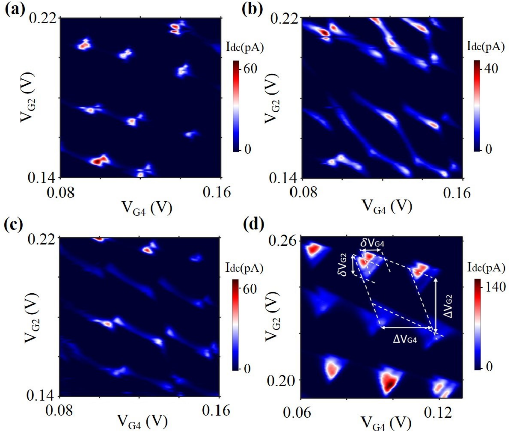
图 3.2 (a)-(c) 当 V_{SD} = 0.5 \text{ mV} 、 V_{G1} = -0.82 \text{ V} 、 V_{G5} = -0.2 \text{ V} 时，在不同中间栅极电压 V_{G3} (0 V, -0.02 \text{ V} , -0.04 \text{ V} ) 下，扫描 V_{G2} 和 V_{G4} 测到的输运相图。(d) 当 V_{SD} = 2 \text{ mV} ， V_{G1} = -0.82 \text{ V} ， V_{G3} = 0.008 \text{ V} ， V_{G5} = -0.17 \text{ V} 时，观测到一组排列整齐的偏压三角形输运相图。
